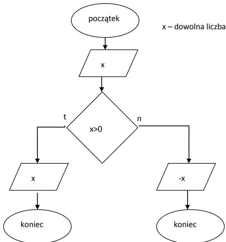
Schemat blokowy – wyznaczenie wartości bezwzględnej z liczby x
